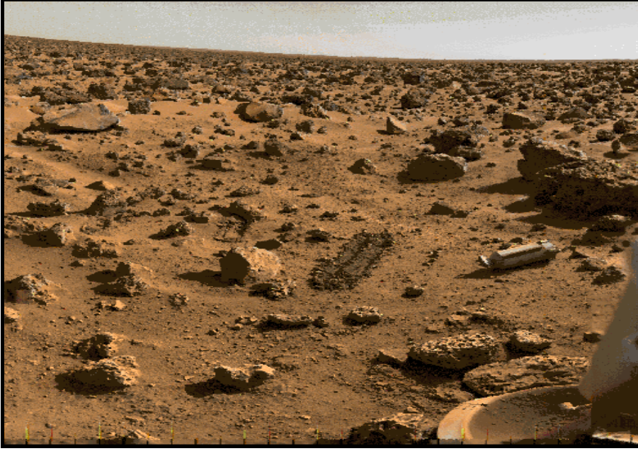
الشكل (8) سطح كوكب المريخ
