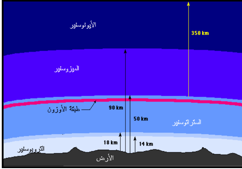
الشكل (2) طبقات الغلاف الجوي
