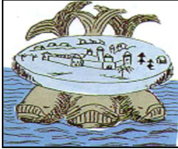
الشكل (28) إعتقد الروس القدامى أن الأرض قرص تحمله ثلاثة حيتان عظيمة
