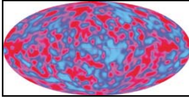
الشكل (36) التوزيع الزاوي للخلفية المايكروية الكونية
