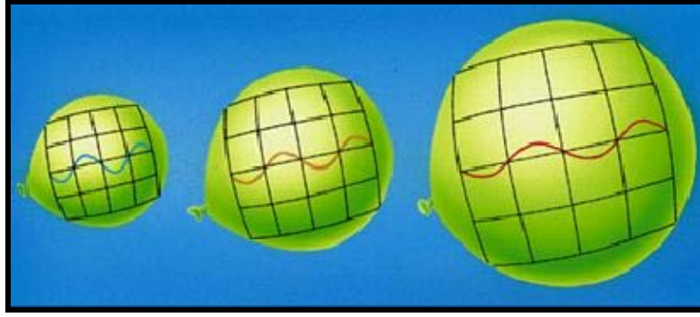
الشكل (32) الازاحة الحمراء للأشعة الكهرمغناطيسية اثناء اتساع الكون
