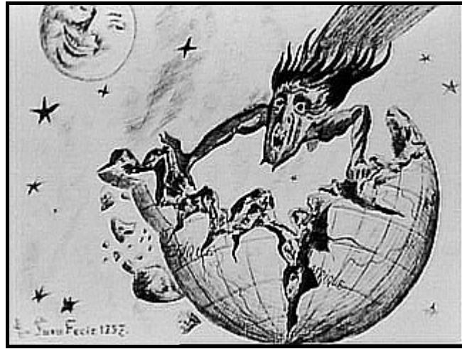
الشكل (14) اعتقد الناس قديما أن المذنبات هي نذير شؤم وشاعت كثيرا حكايات اصطدام المذنبات مع الأرض
