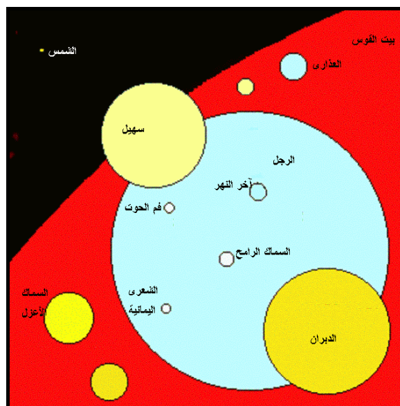
الشكل (19) مقارنة بين الشمس وعدد من النجوم
