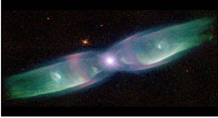
الشكل (18) سديم كوكبي هو مصير أحد الشموس
