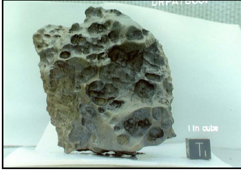
الشكل (16) حجر نيزكي
