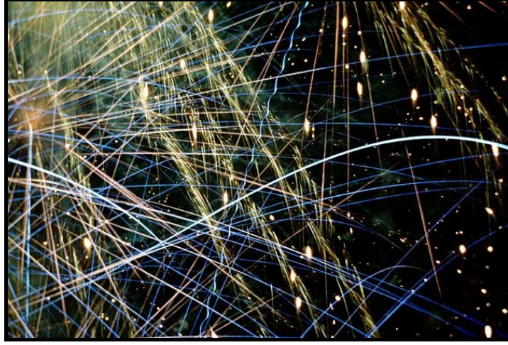
الشكل (15) منظر خلاب مركب من عدة لقطات لشهب البرشاويات
