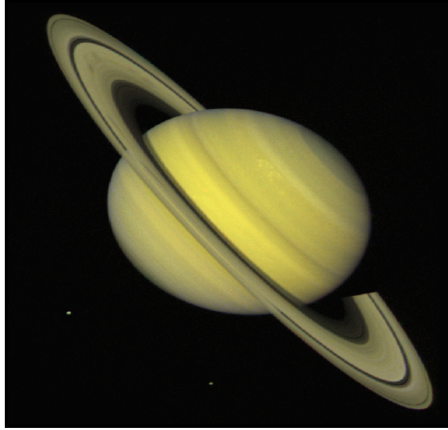
الشكل (12) كوكب زحل ذو الحلقات البهية
