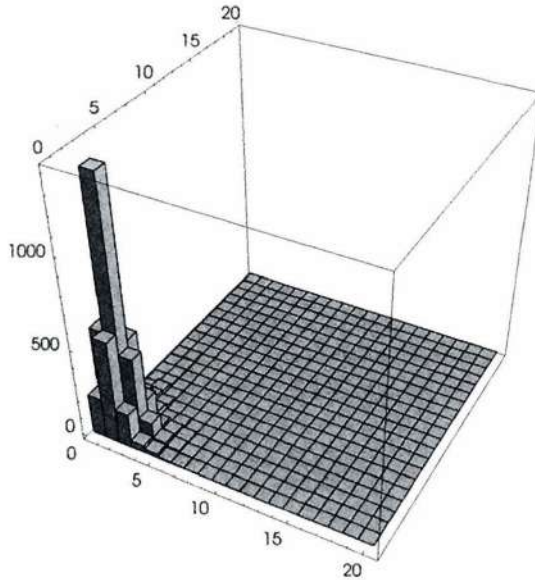
الشكل رقم 13: الجبل الإحصائي النمطي الخالص
