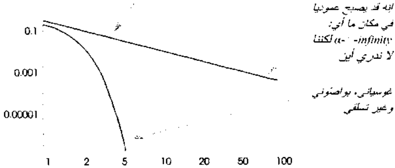
خط مستقيم تسلسلي (انحدار قريب من 1.5) إلى اللانهاية
