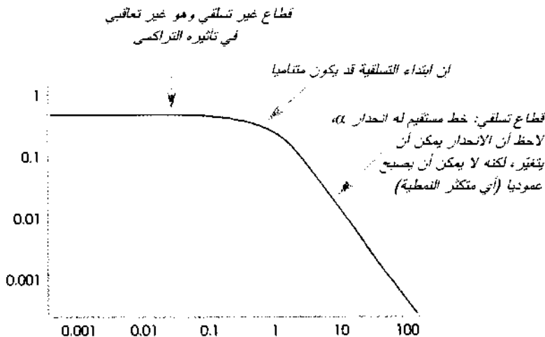
الشكل رقم 15: توزيع نمونجي بأنيال قانون القوة (هنا طالب T)
