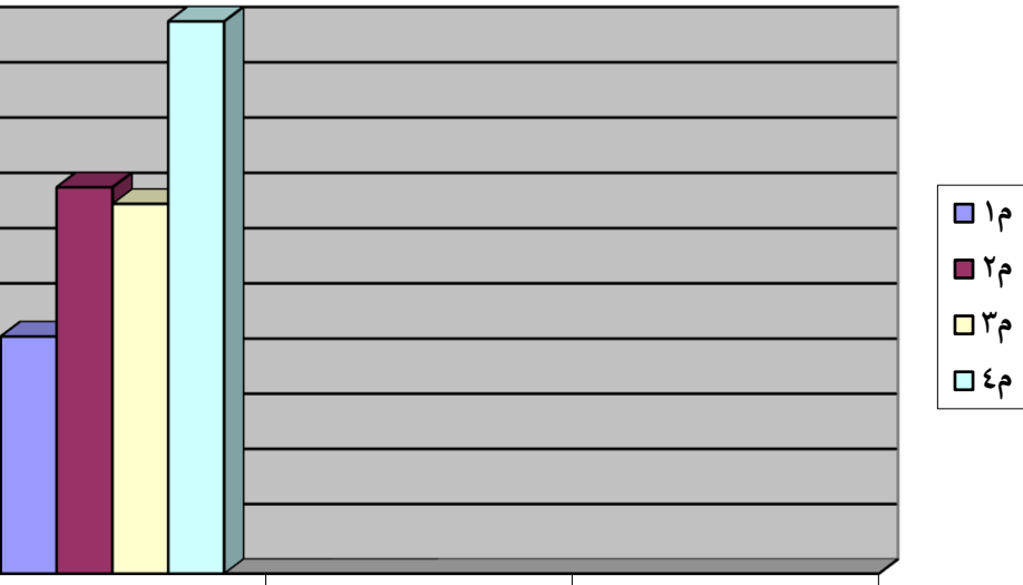
شكل رقم (1) الرسم البياني للفروق للمقاييس الأربعة المعتبرة.
