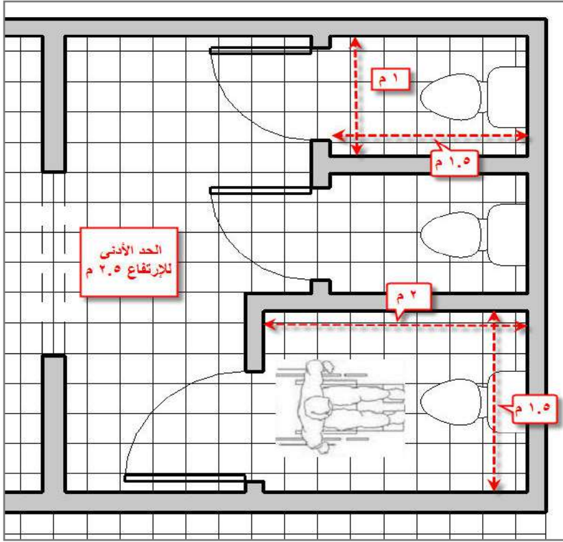
الشكل ٣٥ : أبعاد الحمامات
