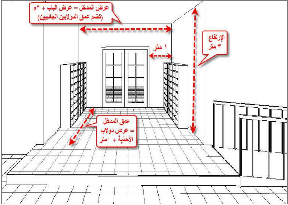
الشكل ١٦ : مواصفات مدخل المصلى
