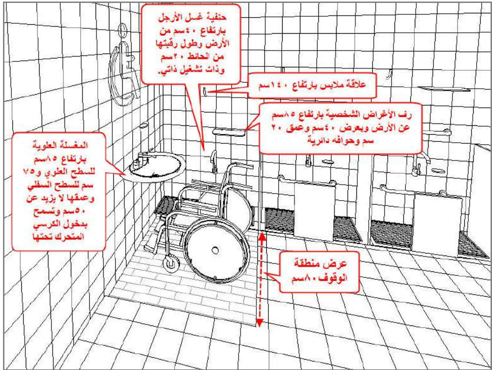
الشكل ٤٣ : موضئ الكرسي المتحرك
