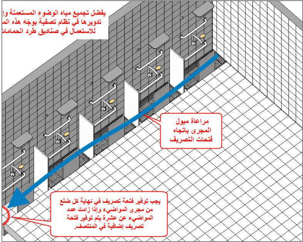
الشكل ٣٨ : ميل المواضع
