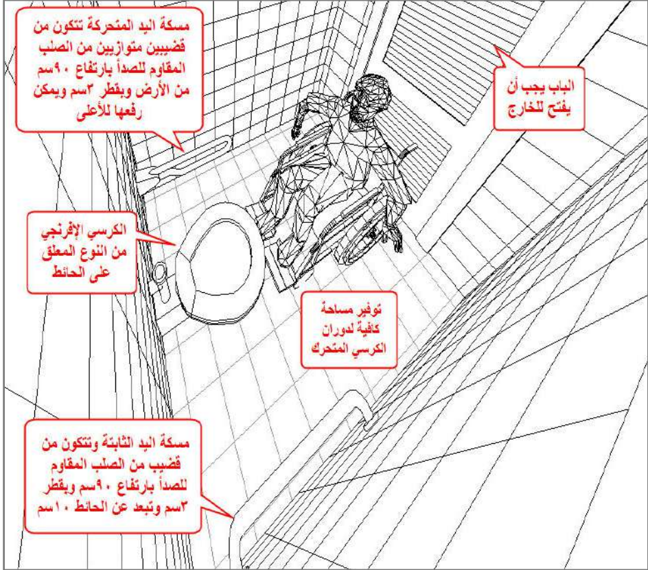
الشكل ٣٧ : حمام ذوي الاحتياجات الخاصة
