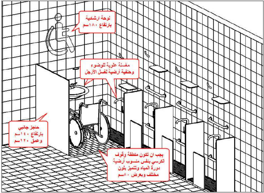
الشكل ٤٢ : موضئ الكرسي المتحرك
