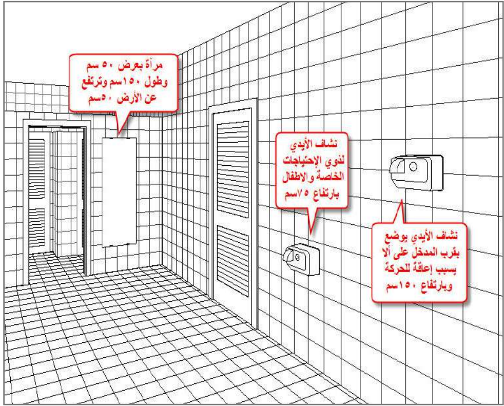
الشكل ٣٤ : ملحقات دورات المياه
