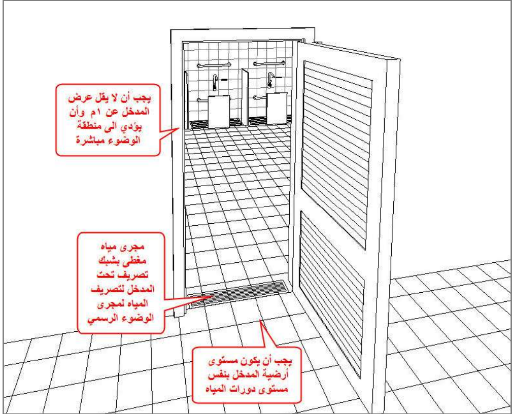
الشكل ٣٠ : مدخل دورة المياه
