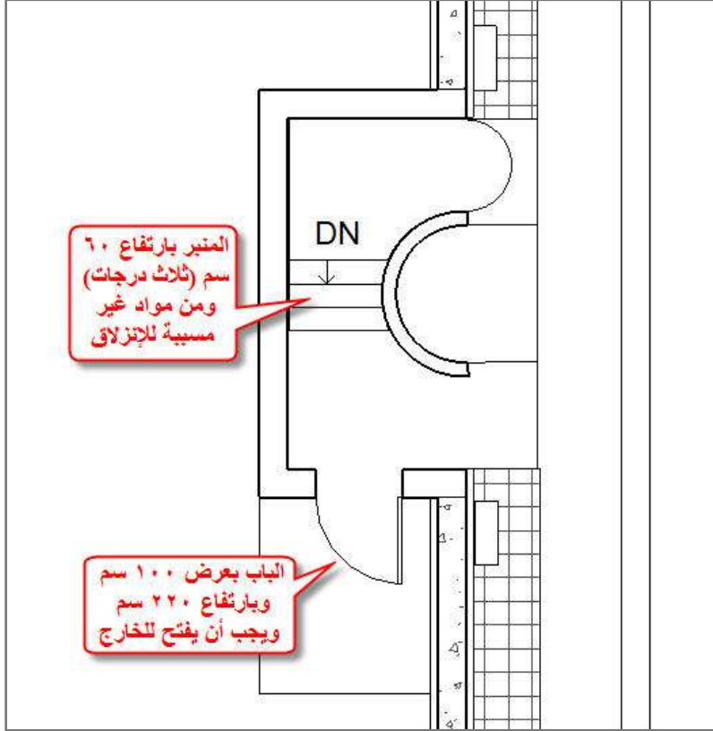
الشكل ٢١ : المنبر و باب المحراب
