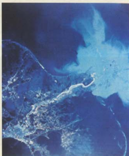
صورة حقيقيه مأخوذه بواسطة الأقمار الصناعية لدلتا أحد الأنهار يصب في البحر دون أن يختلط الماء العذب (باللون الأزرق الفاتح) والمالح (باللون الأزرق الغامق)
