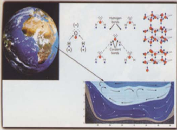
رسم تخطيطي لتباين مياه البحار والمحيطات تباينا رأسيا في صفاتها الطبيعية والكيميائية
