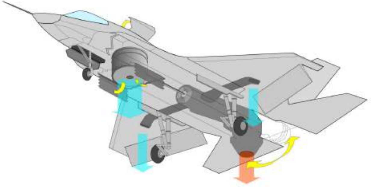
(LiftSystem)الرسم التخطيطي لمكونات نظام الرفع وتدفق الهواء
