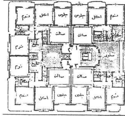
شكل (٢-٣٠) المسقط الأفقى للدور المتكرر عمارة خورى ريمون انتونوس - مدينة (١٩٤١)
